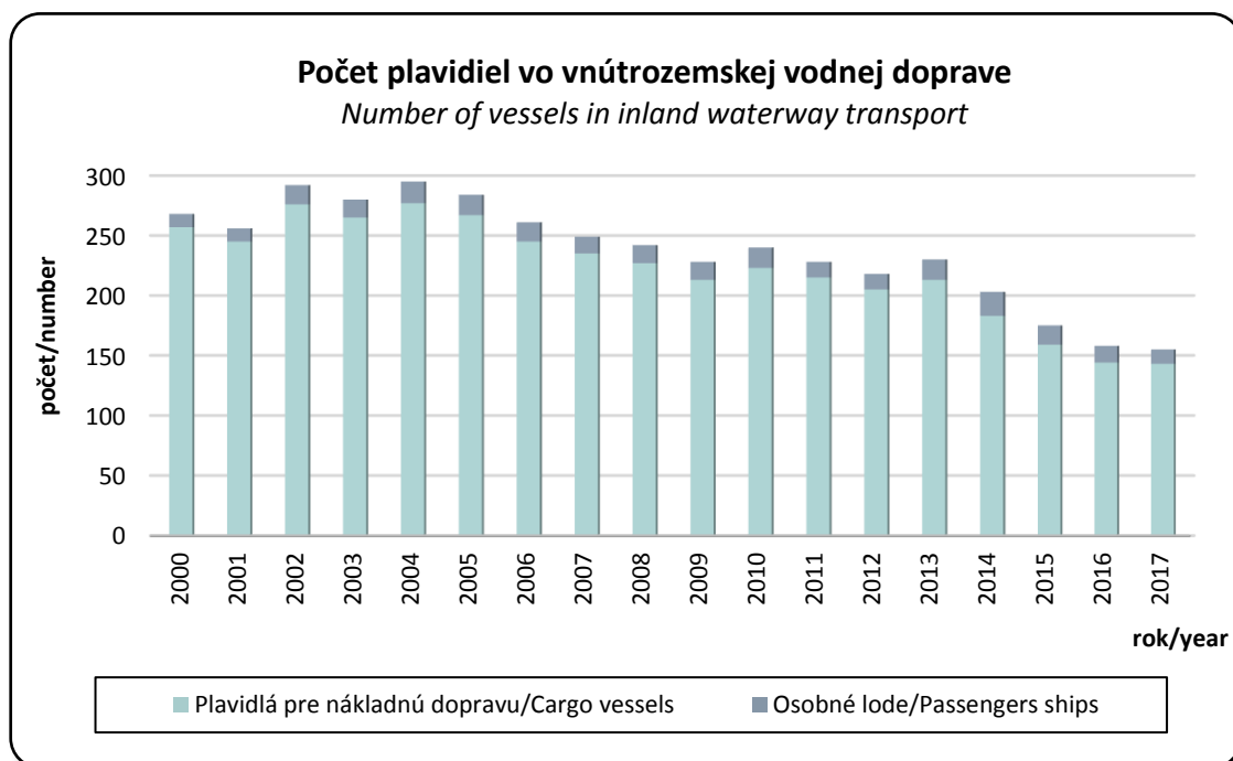
GRAF 8 POČET PLAVIDIEL VO VNÚTROZEMSKÉJ VODNEJ DOPRAVE GRAPH 8 NUMBER OF VESSELS IN INLAND WATERWAY TRANSPORT (GRAFICKÉ ZNÁZORNENIE TABUĽKY 4.3) (GRAPHIC REPRESENTATION OF TABLE 4.3)
