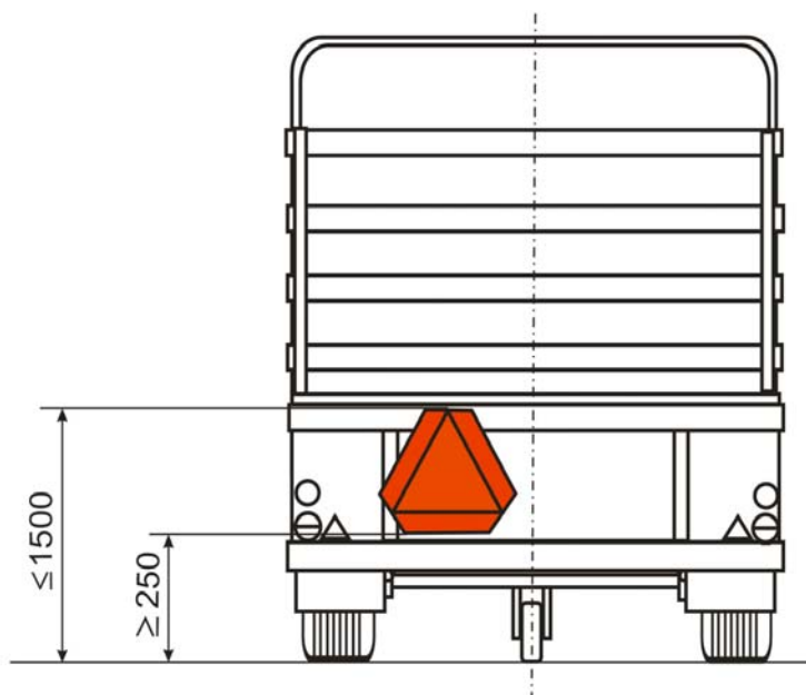
Obr. č. 2 – montáž a umiestnenie podľa predpisu EHK 69 príloha č. 15
