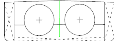
Typ C Konštrukcia nákladného tanku 1 Typ nákladného tanku 1
