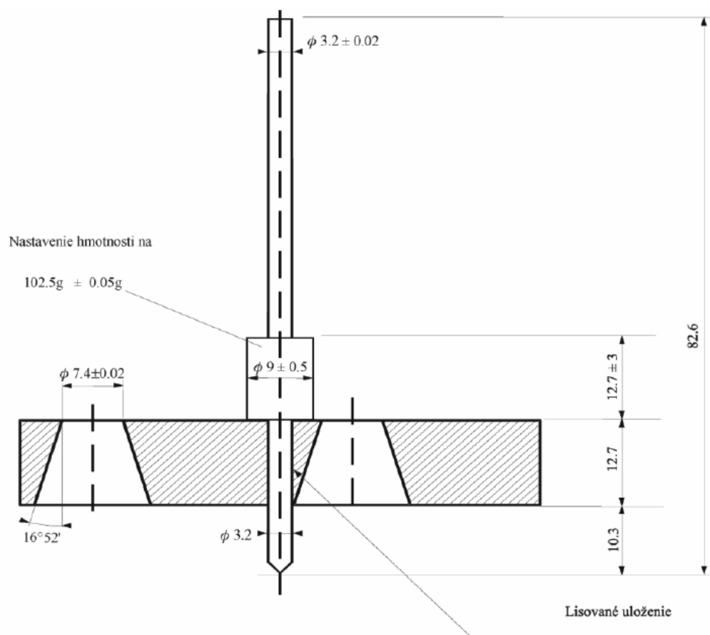
Obrázok 1 - Penetrometer
