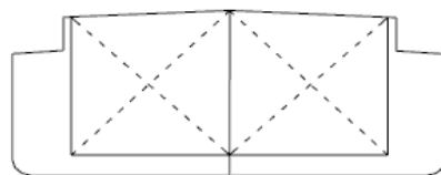
Typ N Konstrukcia nákladného tanku 2,3 a 4 Typ nákladného tanku 1 (aj s hladkou palubou)
