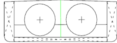
Typ C Konstrukcia nákladného tanku 1 Typ nákladného tanku 1
