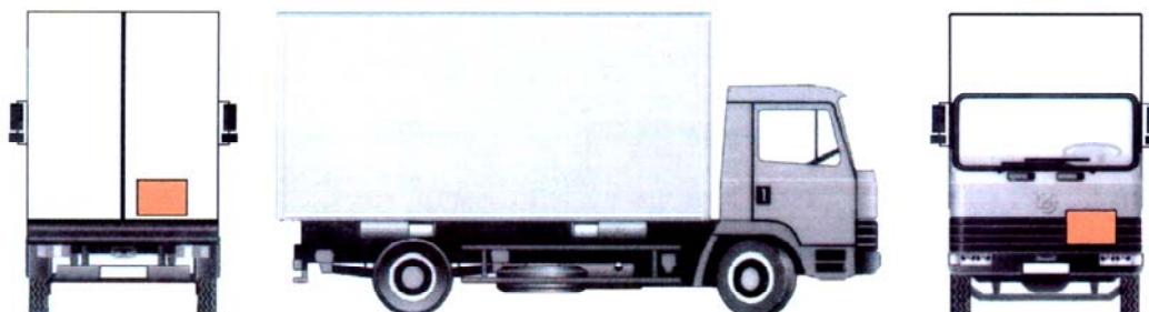
Obrázok č. 1 : Označenie vozidla pri preprave nebezpečných vecí v kusových zásielkach
